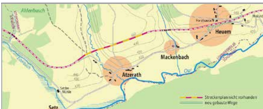
Atzerath-Heuem: Der geplante Streckenverlauf im Bereich Atzerath-Heuem.
